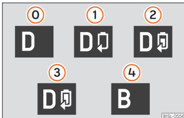
Abb. 136 Im Display des Kombi-Instruments: Anzeige der Rekuperationsstufen.
