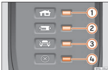
Abb. 158 Am Ladekabel für Netzsteckdosen: Schutzeinrichtung.
