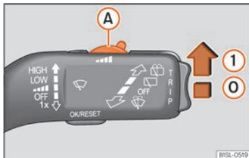
Abb. 85 Scheibenwischerhebel: Regensensor (A) einstellen
