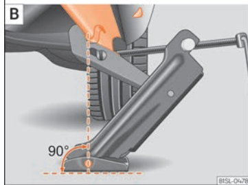
Abb. 36 Längsholm: Wagenheber ansetzen.
