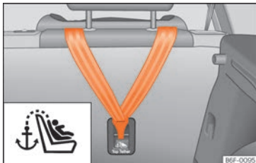
Abb. 25 Rückseite der Rücksitzbank: Halteösen für den Top Tether Haltegurt.
