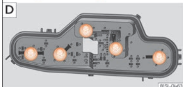
Abb. 53 Rückleuchte: Lampenhalter ausbauen
